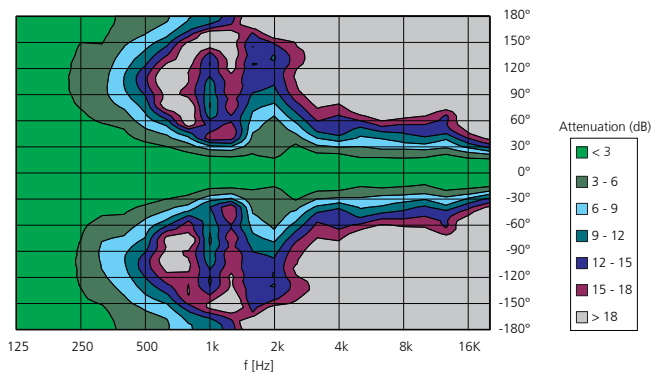
Vertikales Abstrahlverhalten
