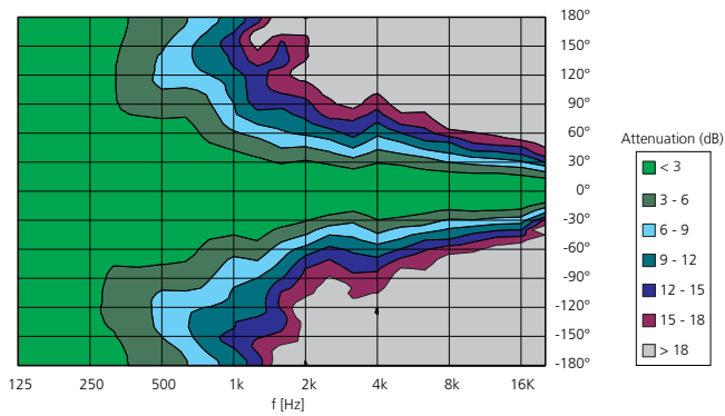
Horizontales Abstrahlverhalten
